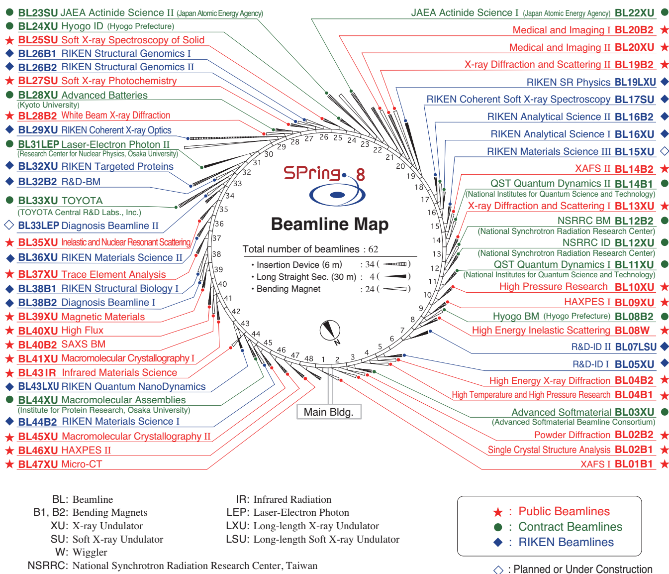
Fig. 2. Beamline map.
